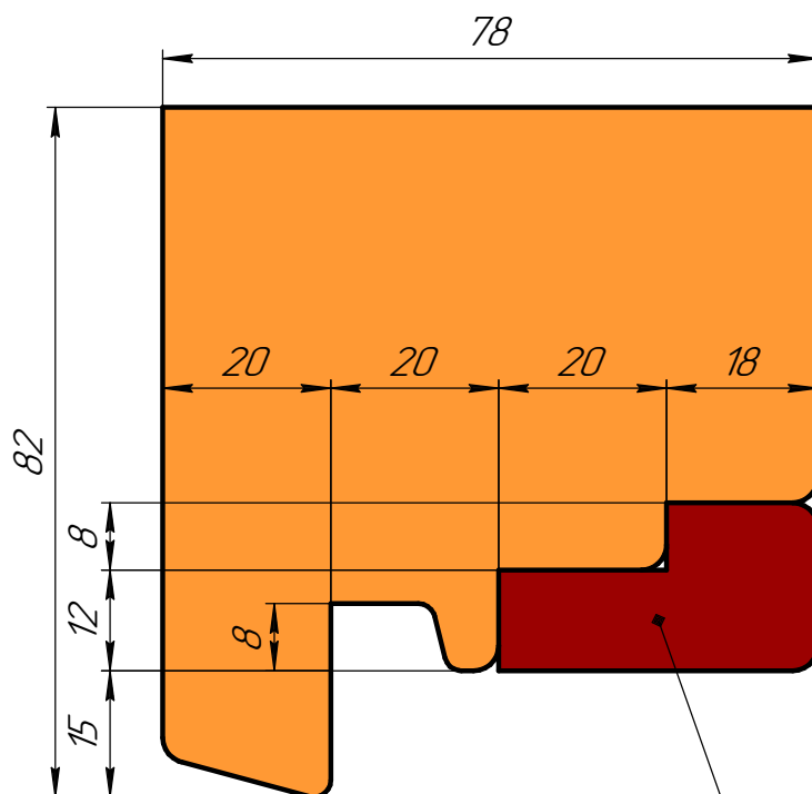
Доборная планка. Тип 2
