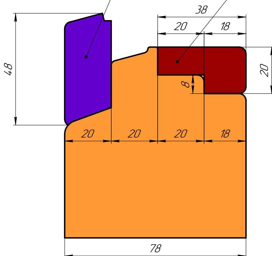
Доборная планка. Тип 2
