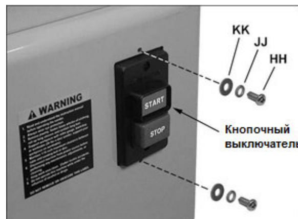
Рис. 13 (однофазная модель)
