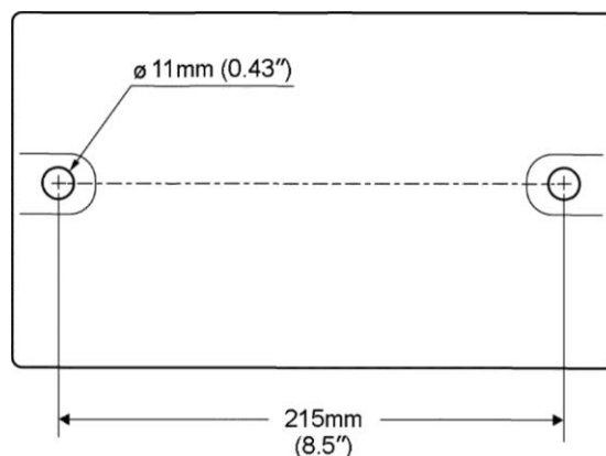
Рисунок 1 Монтажные отверстия.
