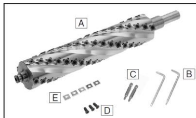
Рис. 19 Компоненты ножевого вала Helical
