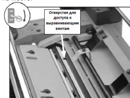
Рис. 17 Отверстия для доступа к выравнивающим винтам в ножевом вале
