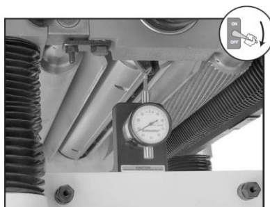
Рис. 23 Использование ротакатора для нахождения НМТ
