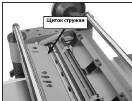
Рис. 27 Щиток стружки и фиксирующие болты
