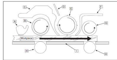
Рис. 2 Внутренние компоненты
