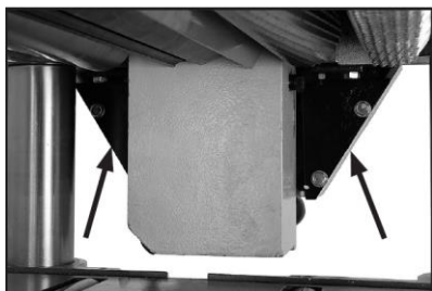
Рис. 21 Задние щитки крышки звездочек
