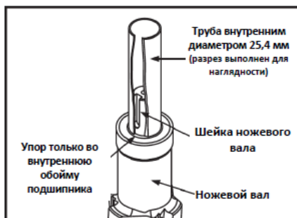
Рис. 30 Установка подшипника
