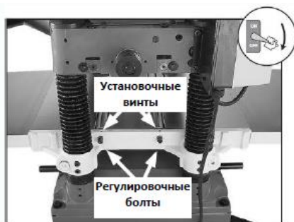
Рис. 14 Регулировка высоты опорных роликов
