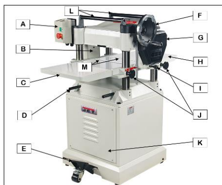
Рис. 1 Общие обозначения
