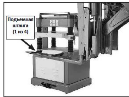
Рис. 3 Подъем с помощью погрузчика
