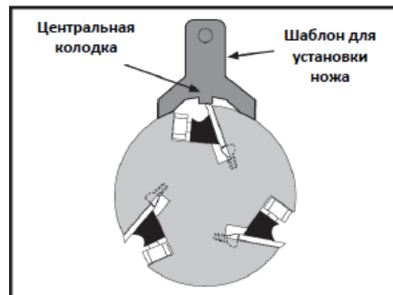
Рис. 16 Правильное положение шаблона для установки ножа
