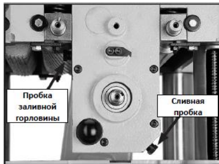
Рис. 23 Расположение пробки заливной горловины и сливной пробки
