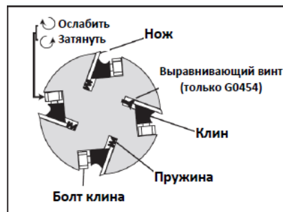
Рис. 15 Компоненты ножевого вала
