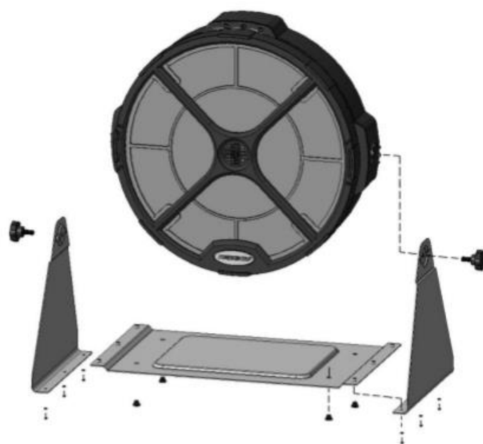
Рисунок 8-1: Сборка
