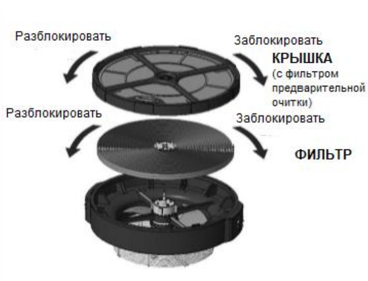
Рисунок 8-4: Замена фильтра
