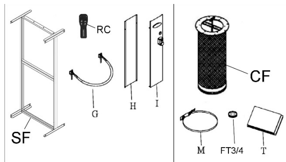
Рисунок 2: Содержимое ящика № 2 и №3
