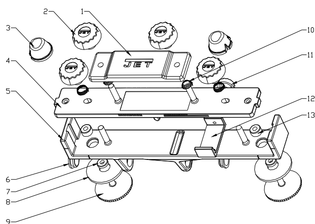
PCJ-1 Приспособление для заточки строгальных ножей
