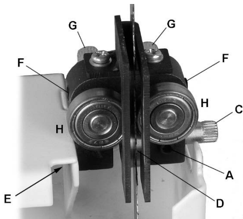
Рис. 26 Нижние направляющие полотна
