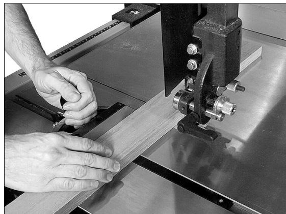
Рис. 42: поперечный распил
