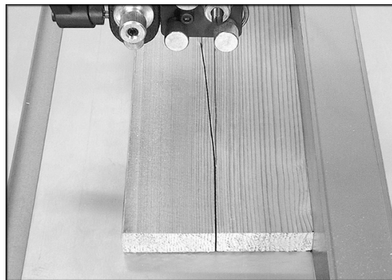
Рис. 45: смещение полотна
